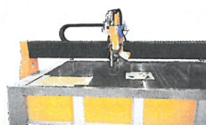
Wasserstrahlschneidemaschine Powerjet 3D Fotos: Firma
